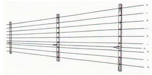
Clôture électrique verticale (source : Fontaine et al. , 2002).
