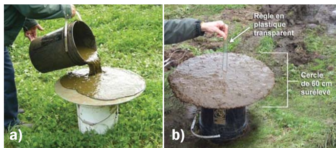
Figure 3 : Mesure de l'affaissement du lisier.
