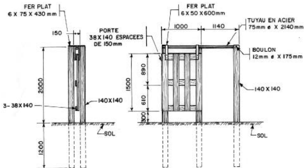
DETAIL DE LA CLÔTURE
