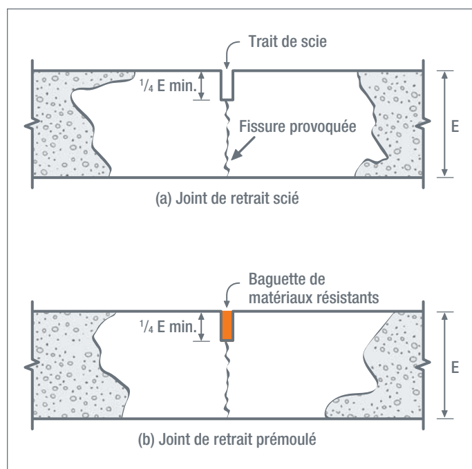
Figure 6 - Joint de retrait scié et prémoulé
