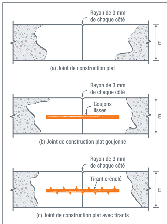
Figure 7 - Différents joints de construction
