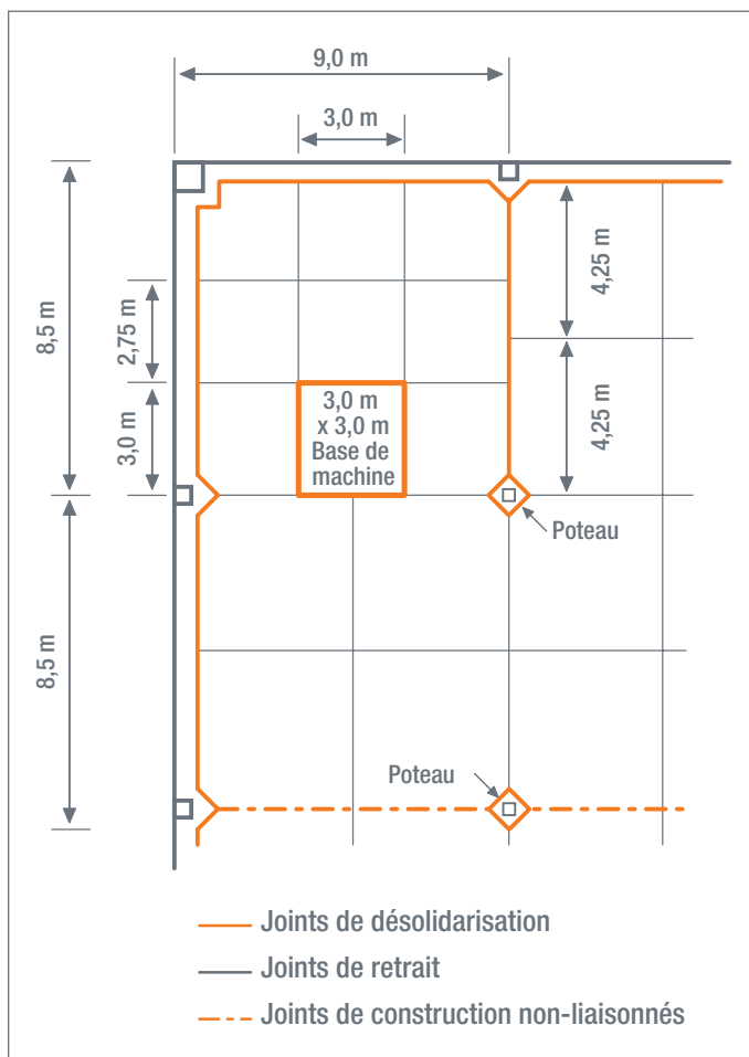
Figure 4 - Disposition caractéristique des joints d'une dalle
