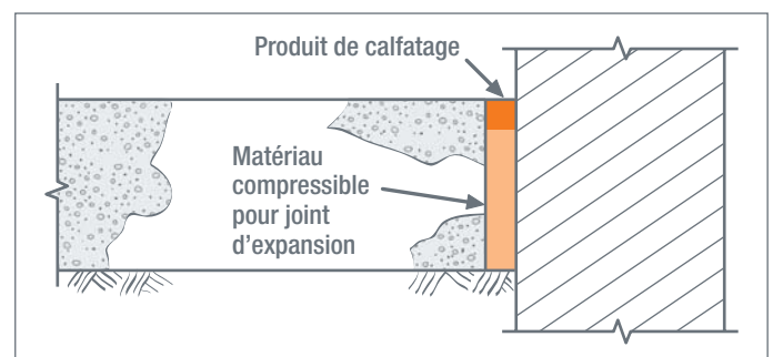
Figure 5 - Joint de désolidarisation
