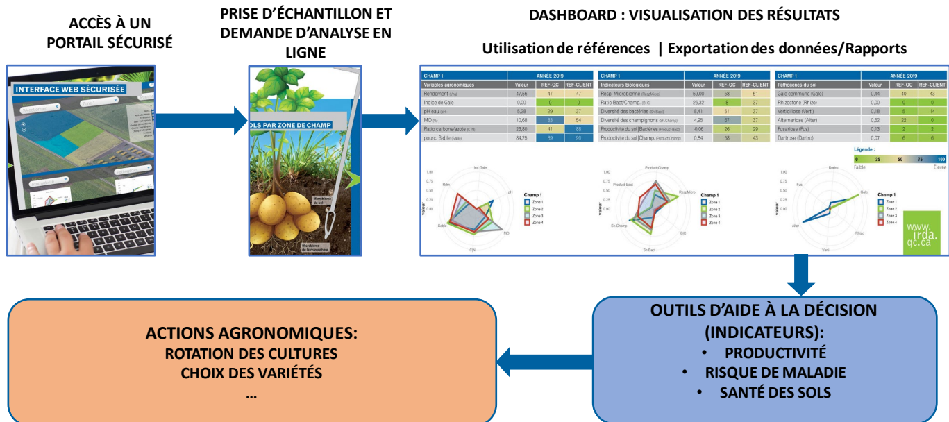
Figure 1 : Maquette du développement et des fonctions de l'application web.
