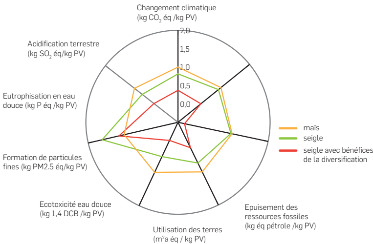
Figure 2 – Impacts environnementaux de 1kg de seigle produit au Québec calculé avec des limites de système standard ou étendues, en comparaison du maïs ACV de l'utilisation du seigle en alimentation porcine
